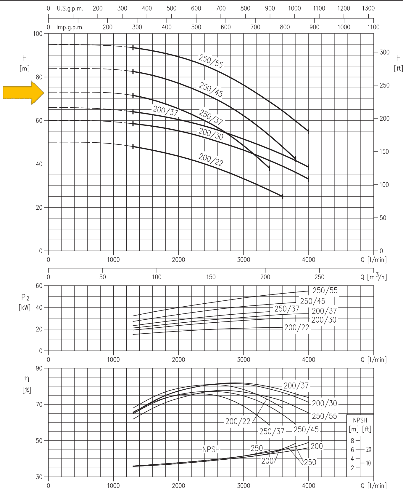
COURBES DE PERFORMANCE SÉRIE 3L 80 à 2900 min -1 (selon ISO 9906 Annexe A)
