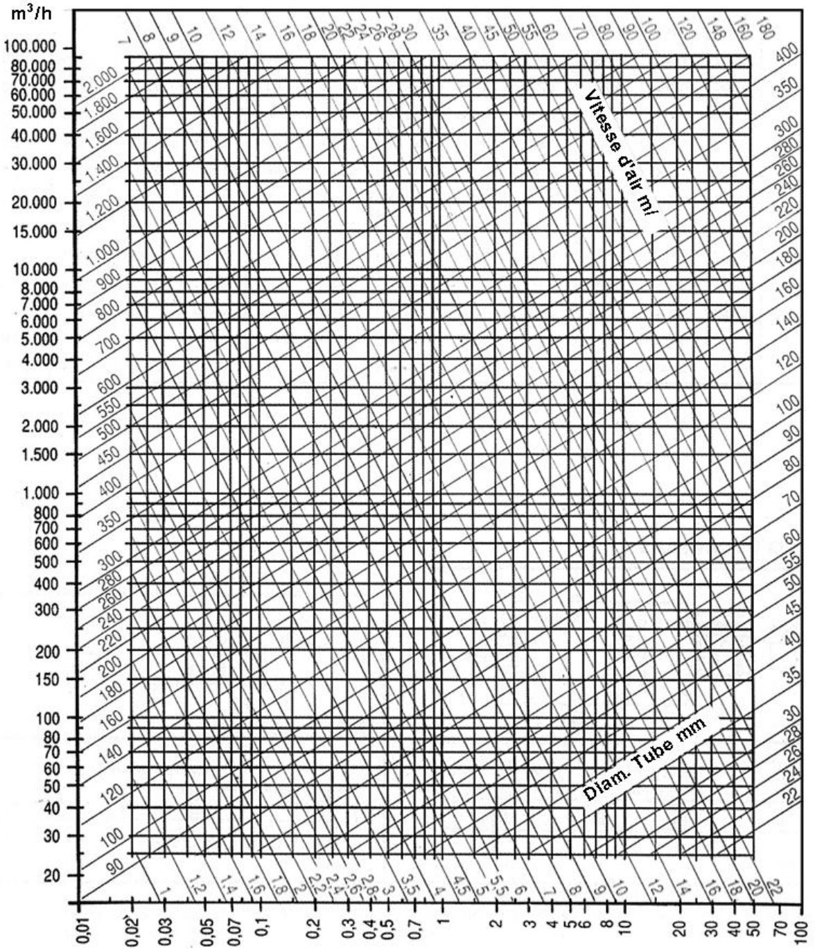
Perte de charge en mm Ce par m de conduit.
